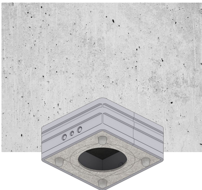
Boîtier d'encastrement pour plafonds / murs en béton:
